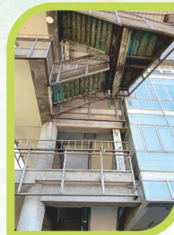
鐵件除鏽及周邊修繕工程進行前，饒平館及逃生梯現況
